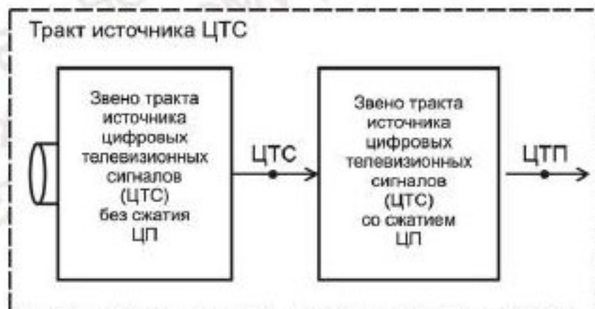
Рисунок 2 — Звенья тракта источника цифровых телевизионных сигналов
