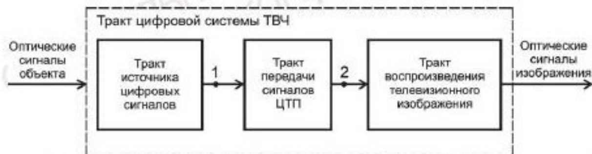
Рисунок 1 — Звенья тракта цифровой системы телевидения высокой четкости
